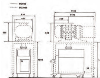
DD605/DD2005
