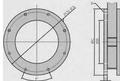
JIS Flange
