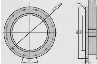
NW Flange
