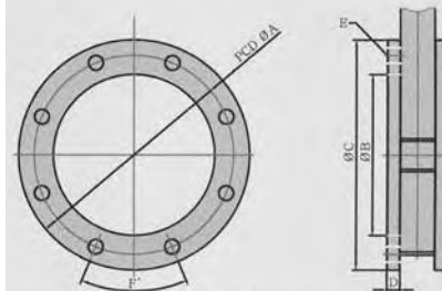
ANSI Flange
